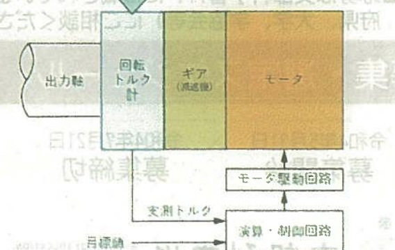
図2：トルクアクチュエータの原理図
